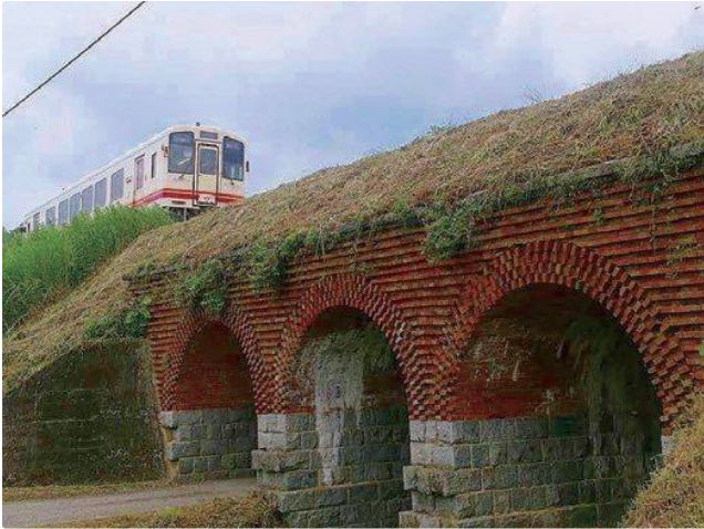
1895년 준공한 우치다 3연 교량
